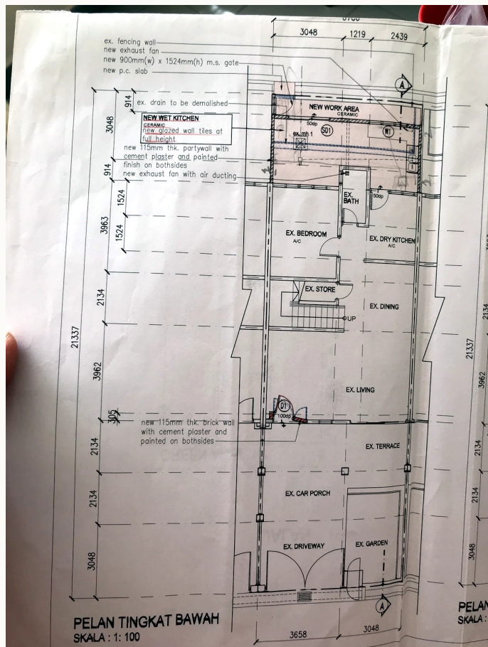
底层平面图
